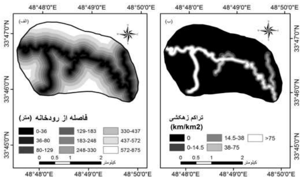
شکل ۴. نقشه (الف) فاصله از رودخانه و (ب) تراکم زهکشی منطقه مطالعاتی Fig. 4. Map of (a) distance from the river and (b) drainage density of the study area
