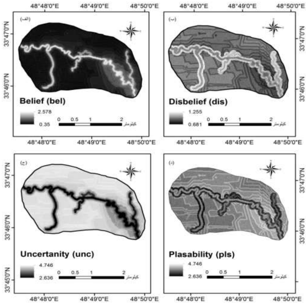
شکل ۶. نقشه‌های حاصل از مدل EBF از (الف) bel، (ب) dis، (ج) unc و (د) pls در منطقه مطالعاتی Fig. 6. Maps resulting from the EBF model (a) bel, (b) dis, (c) unc and (d) pls in the study area
