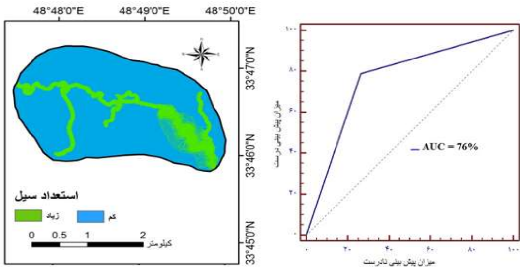
شکل ۷. (الف) نقشه استعداد سیل حاصل از مدل EBF و (ب) منحنی ROC Fig. 7. (a) Flood susceptibility map resulting from EBF model and (b) ROC curve
