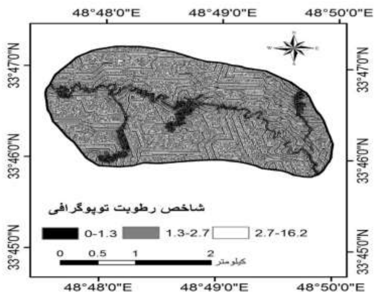
شکل ۵. نقشه شاخص رطوبت توپوگرافی منطقه مطالعاتی Fig. 5. Topographic humidity index map of the study area
