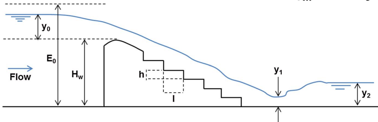
شکل ۱. پارامترهای هندسی و هیدرولیکی مؤثر بر اتلاف انرژی جریان Fig 1. Geometrical and hydraulic parameters affecting flow energy loss
